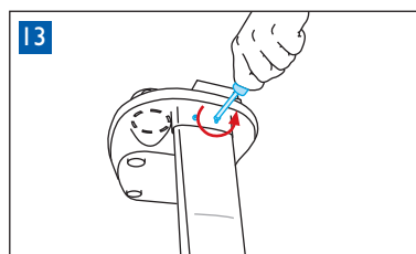
Dévissez les 2 vis tenant le tube rigide.
